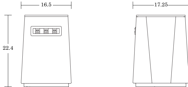
Power Module / QPM
